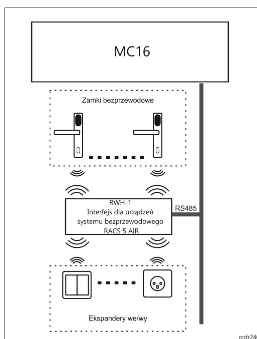
Podłączenie urządzeń systemu RACS 5 AIR do kontrolera dostępu MC16
