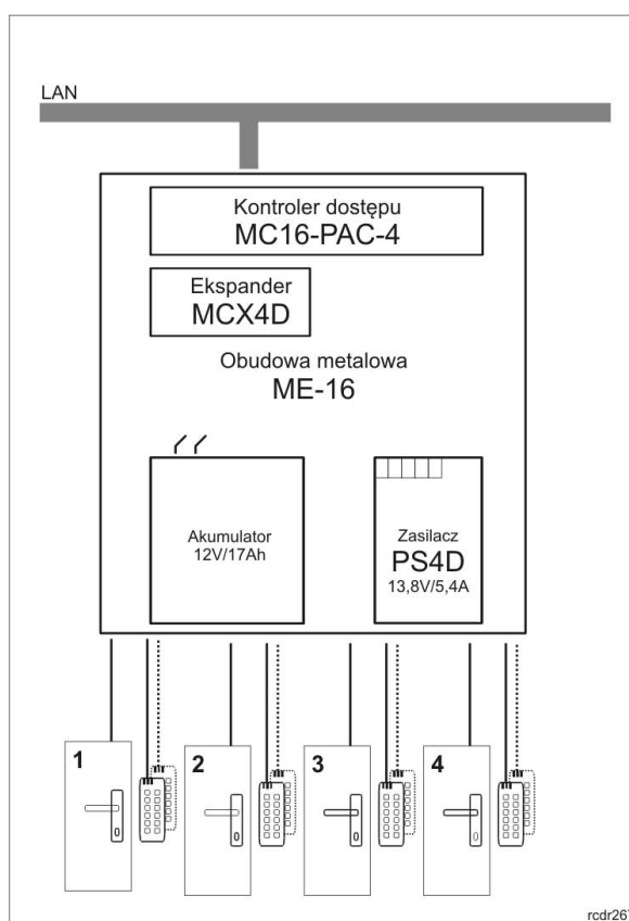
Obsługa 4 przejść z wykorzystaniem kontrolera MC16-PAC-4 i ekspandera MCX4D
