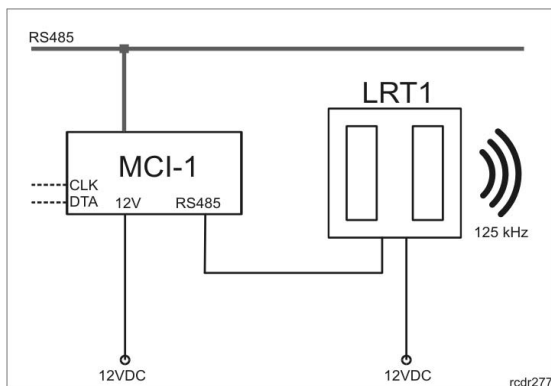
Wykorzystanie interfejsu MCI-1 do podłączenia czytnika dalekiego zasięgu LRT-1
