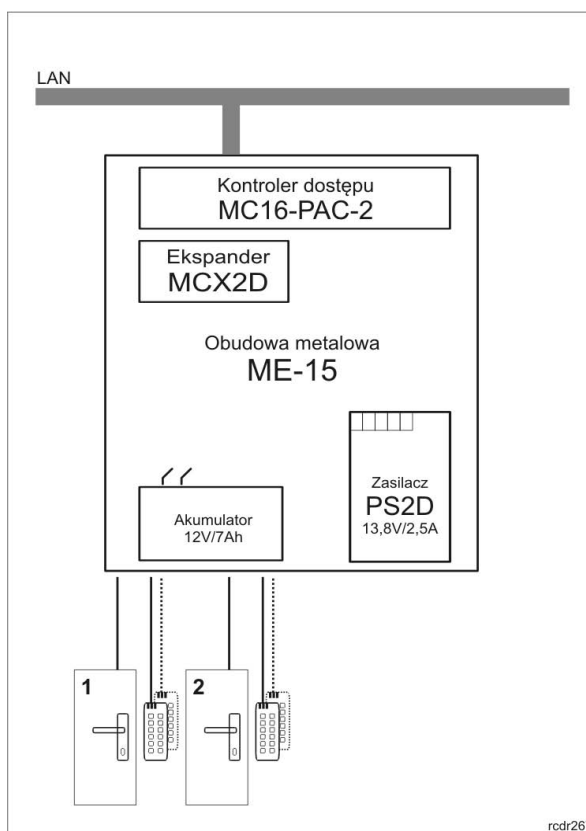
Obsługa 2 przejść z wykorzystaniem kontrolera MC16-PAC-2 i ekspandera MCX2D
