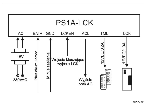
Moduł zasilania PS1A-LCK
