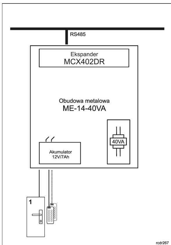
Obsługa 1 przejścia dwustronnego z czynnikiem Wieganda i ekspanderem MCX402DR
