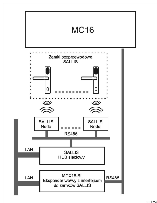
Podłączenie zamków bezprzewodowych serii SALLIS do kontrolera dostępu MC16
