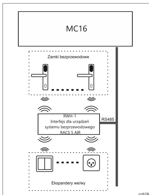
Współpraca kontrolera MC16 z urządzeniami bezprzewodowymi systemu RACS 5 AIR
