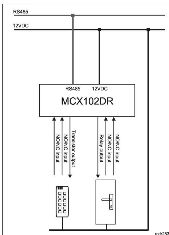
Obsługa przejścia jednostronnego z czujnikiem Wieganda i ekspanderem MCX102DR
