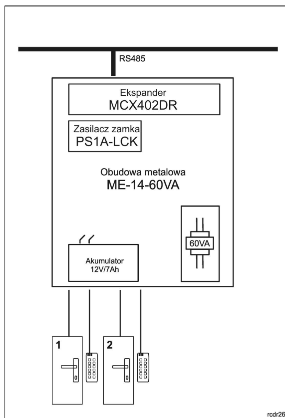
Obsługa 2 przejść jednostronnych z czynnikiem Wieganda, ekspanderem MCX402DR oraz modulem zasilania PS1A-LCK
