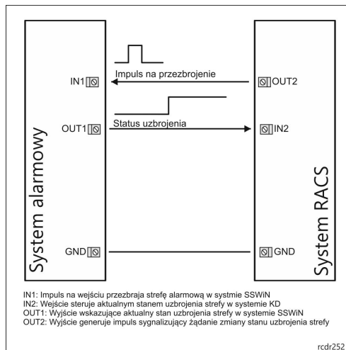
Integracja sprzętowa z systemem alarmowym
