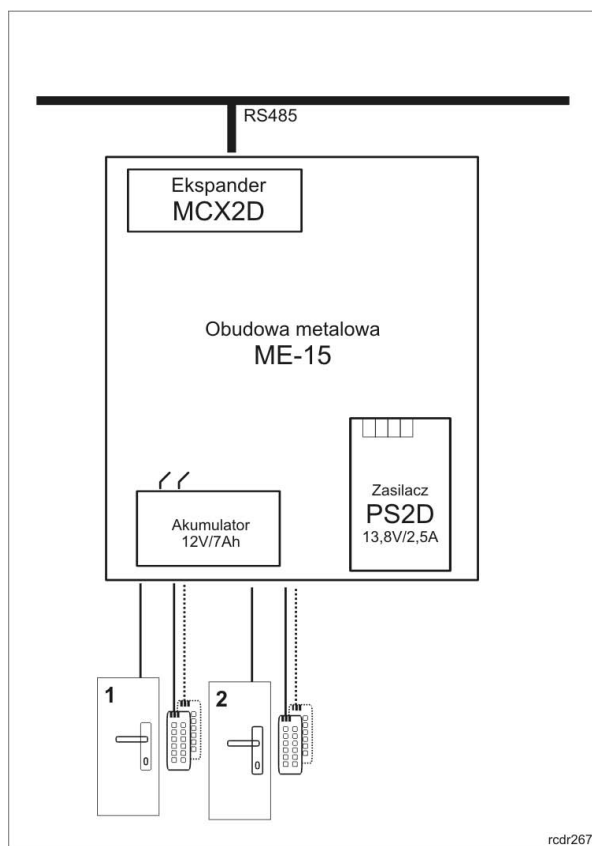
Rozszerzenie o 2 przejścia z czynnikiem MCT
