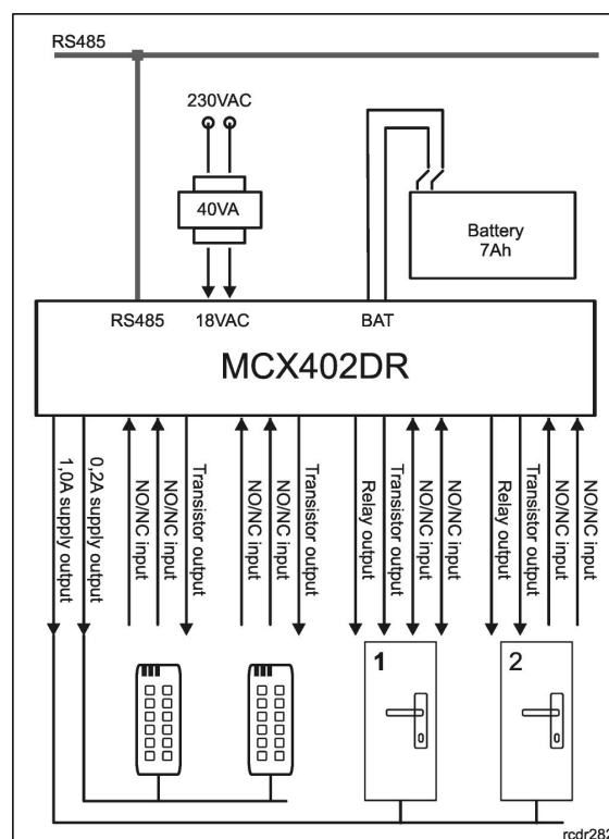
Obsługa przejścia dwustronnego z czytnikami Wieganda i ekspanderem MCX402DR
