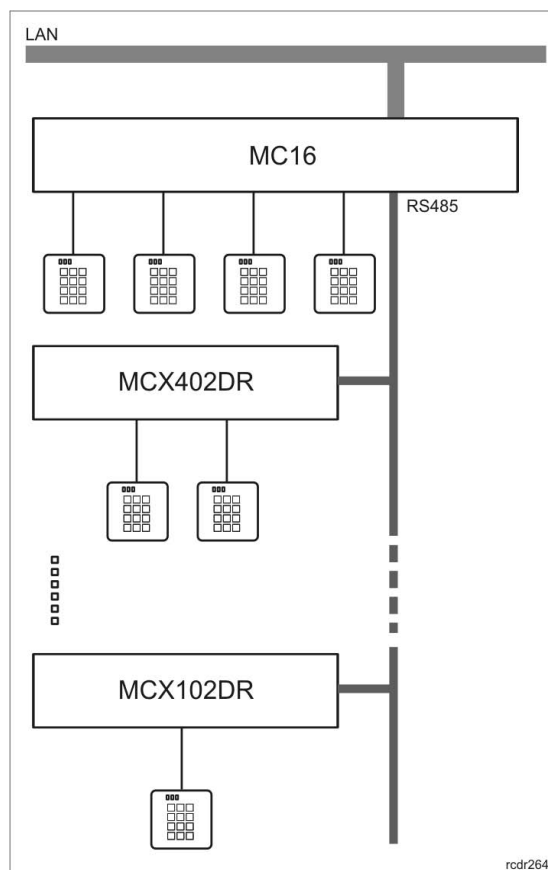
Możliwości podłączenia czytników Wieganda do kontrolera MC16
