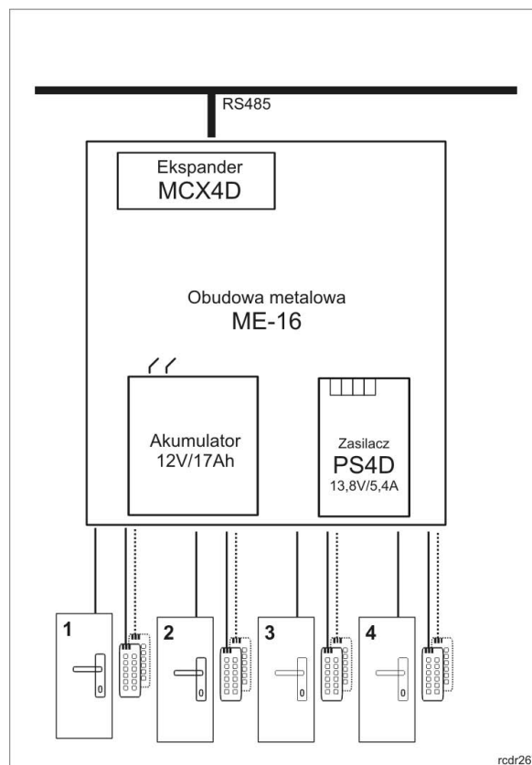
Rozszerzenie o 4 przejścia z czynnikiem MCT
